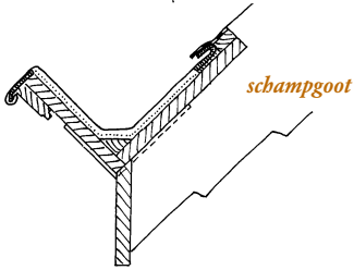
bakgoot
