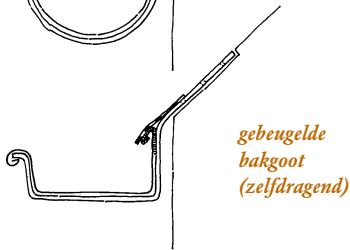
mastgoot (zelfdragend)
